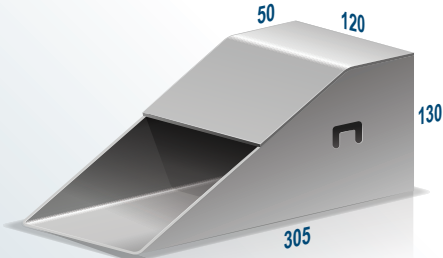
AK1 STANDARD LAYBACK
